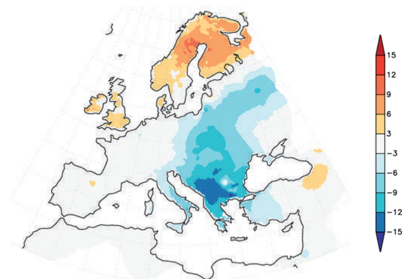
図2 | 2017年1月7～11日の5日間にわたるヨーロッパにおける日平均気温の平年値からの偏差(平年差)。出典: World Weather Attribution (2021年10月27日にアクセス)
