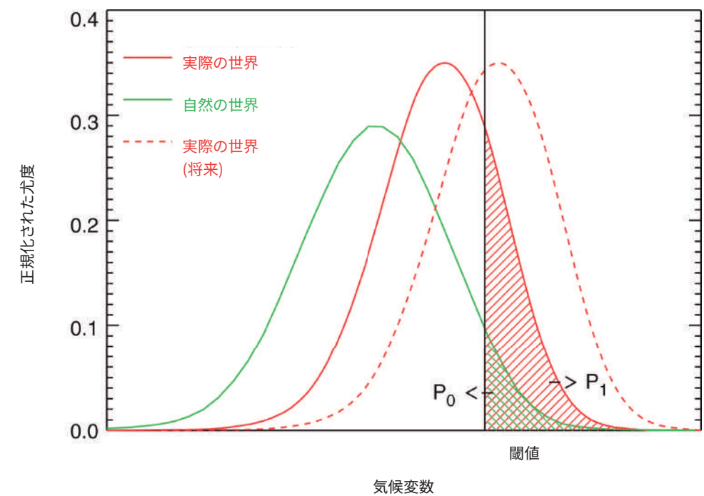
図1 | イベント・アトリビューション研究の例 (Stott et al., 2016)。2つの曲線は日々の気温などの気候変数を示している。平均気温は発生確率が最も高い(曲線の頂点)一方で、極端な気温(曲線の両端にある高温と低温)の発生確率は最も低い。緑の曲線は、それらの気温が「人為影響による温暖化のない産業革命以前の世界」で発生した確率を表している。赤の曲線は現在の地球における発生確率である。閾値は、極端現象(この例では非常に暑い日)の発生時に設定される。網掛け部分の面積の大きさを比べると、現代社会でどの程度現象が発生しやすくなったかが分かる。点線は、将来、気象が今後さらにどう変化するかを示している(この場合、現在の気候の下での非常に暑い日は、将来の気候においては相対的に涼しい日になる可能性を示唆している)。
